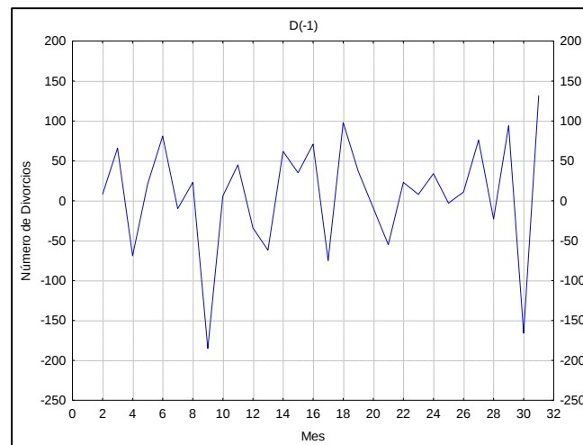
Figura 28. Gráfico de diferenciación a la serie de tiempo.
