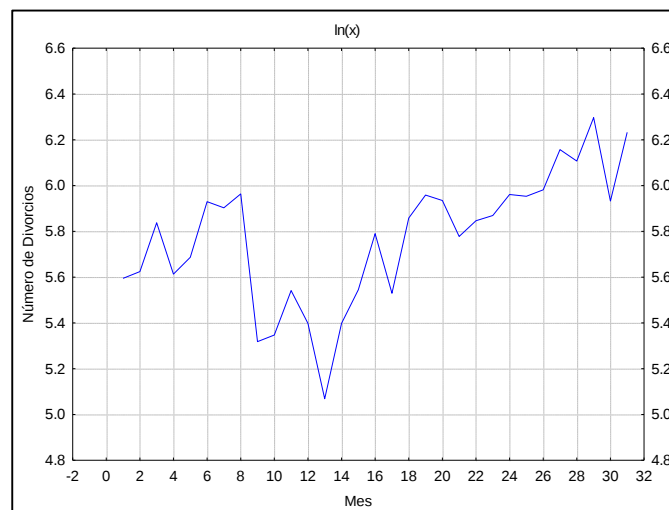
Figura 29. Gráfico de logaritmo natural a la serie de tiempo.
