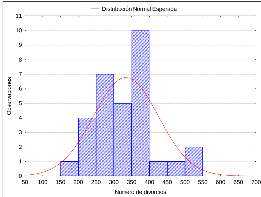
Figura 27. Histograma de la serie de tiempo del número de divorcios por año en Xalapa, Ver.
