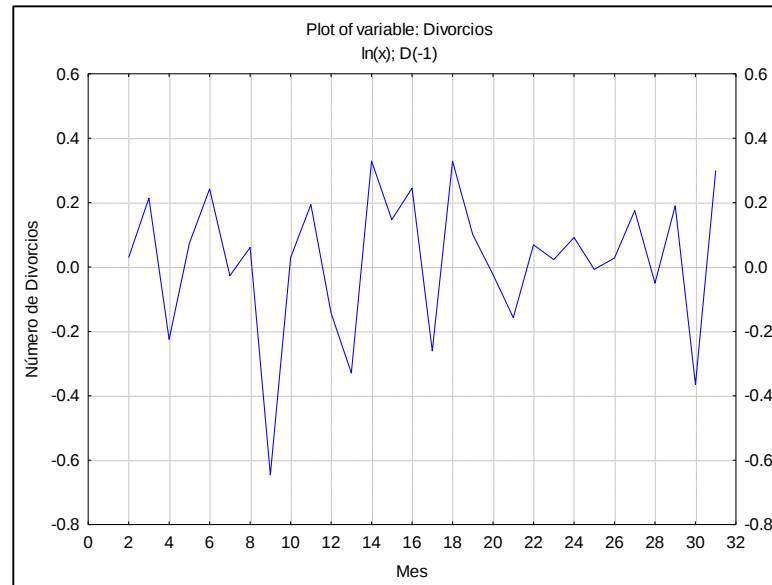
Figura 30. Gráfico de logaritmo natural y diferenciación a la serie de tiempo.
