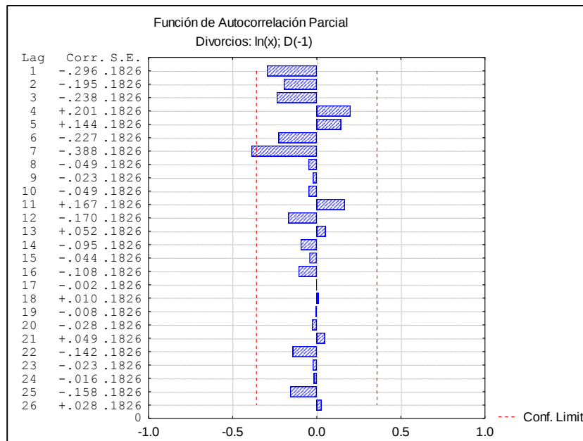
Figura 32. Gráfico de función de autocorrelacion parcial de la serie estacionarizada
